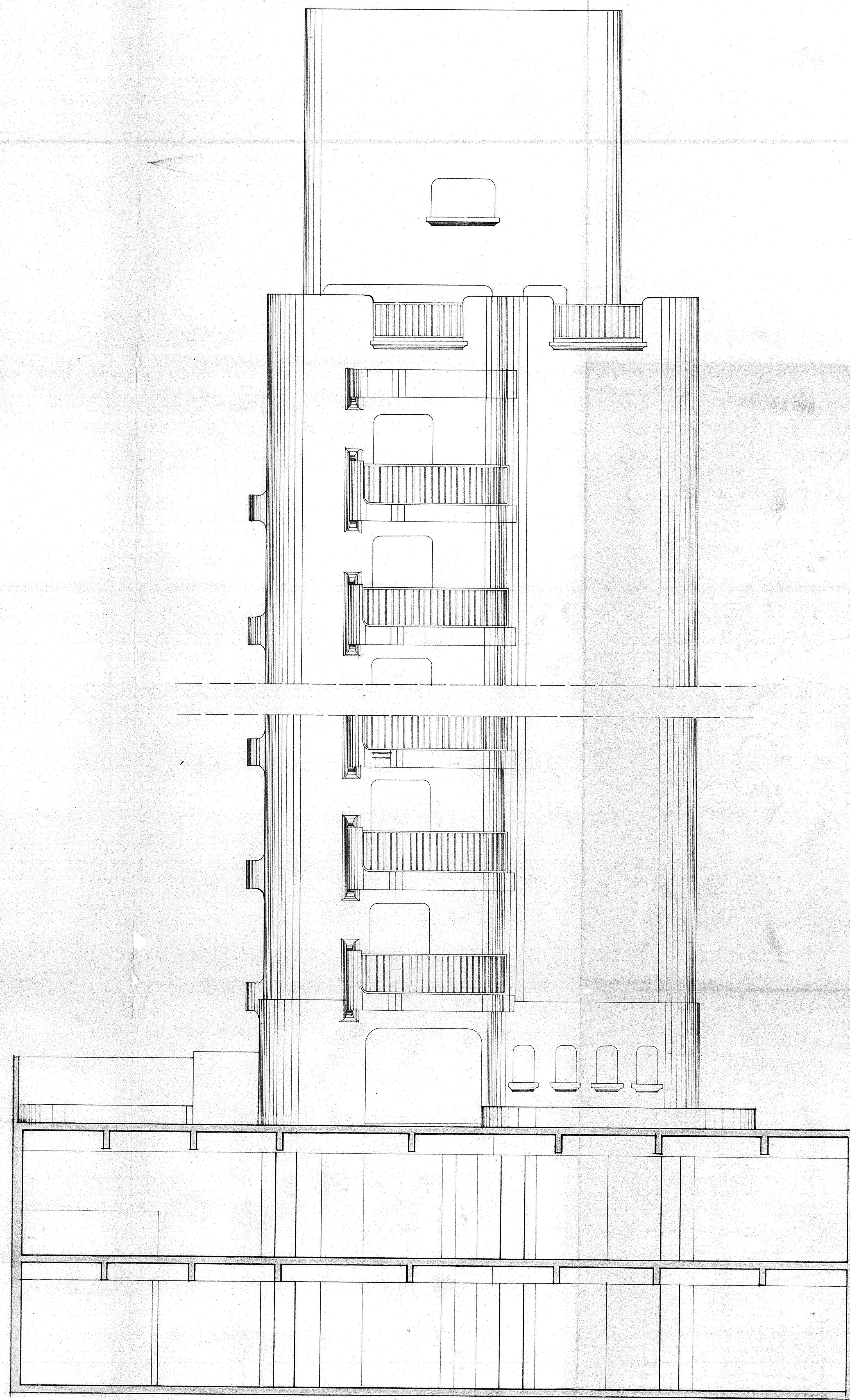
FACHADA POSTERIOR
