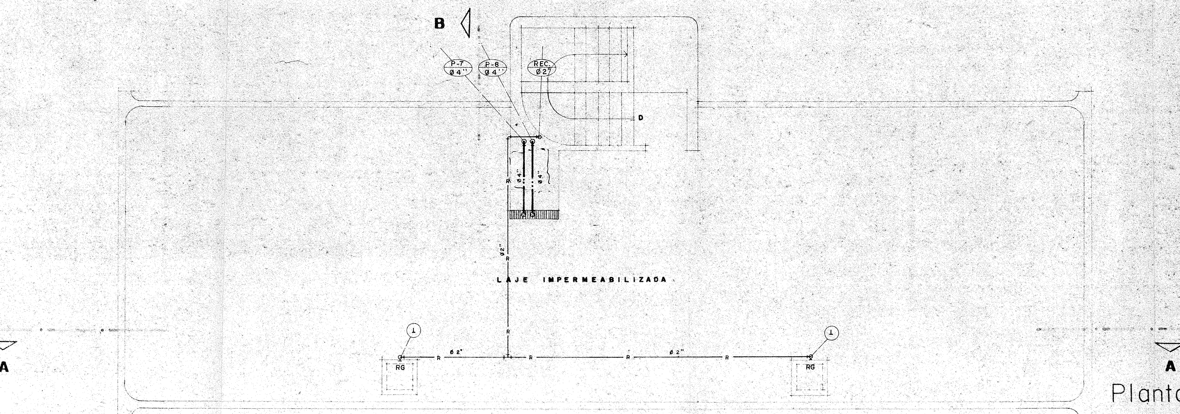
Planta - Barrilete
