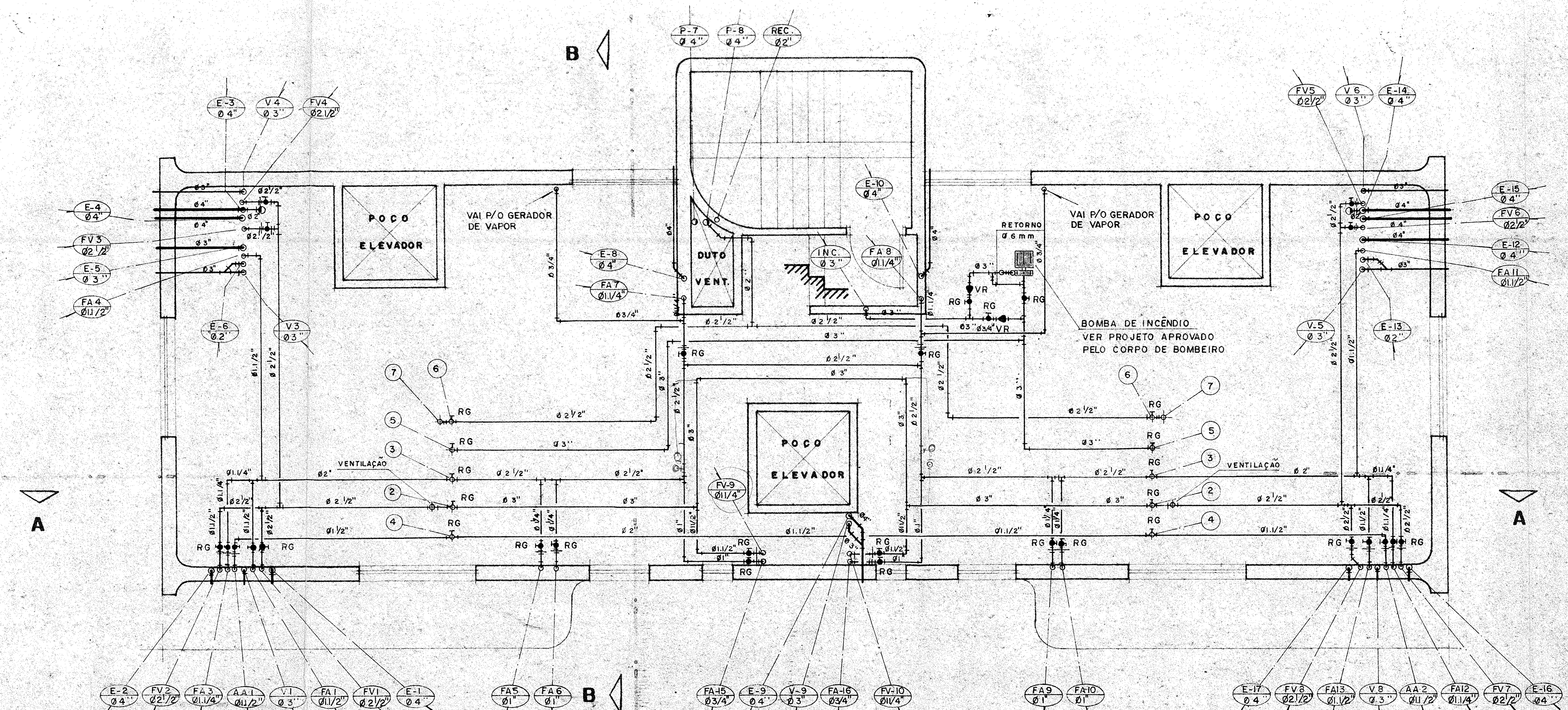
Planta - Barrilete
