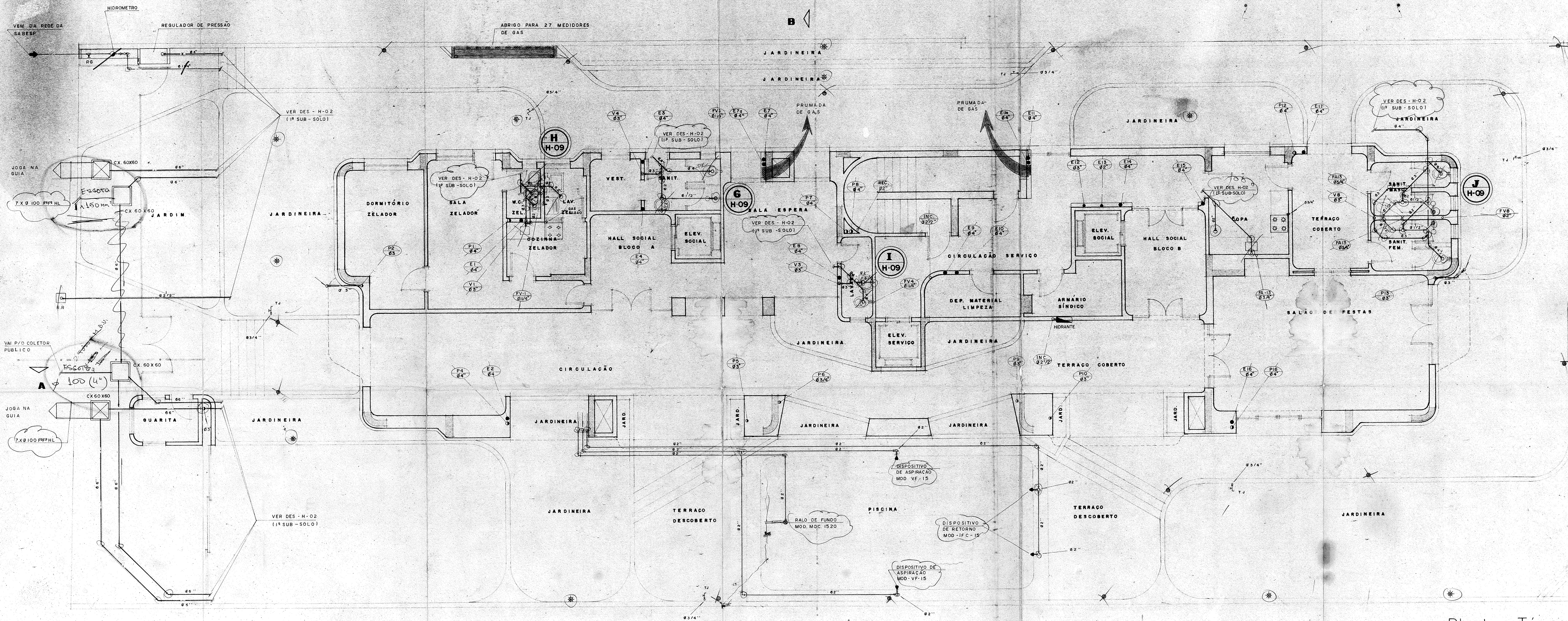
Planta - Térreo
